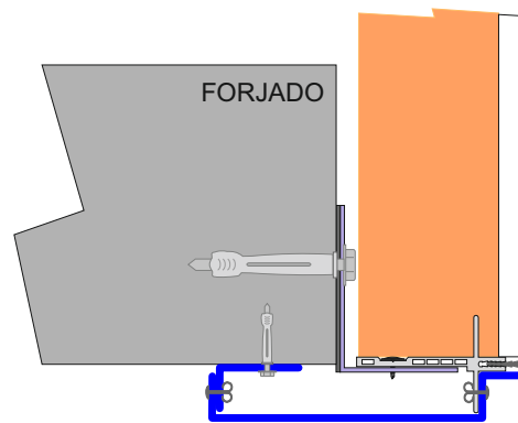
Remate INFERIOR Metálico
