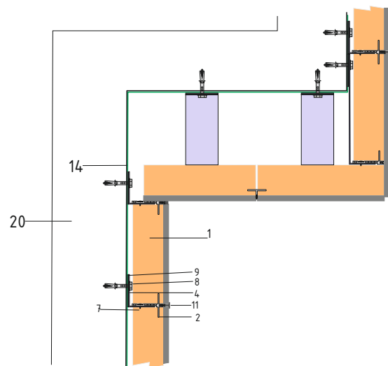
COUPE TRANSVERSALE
