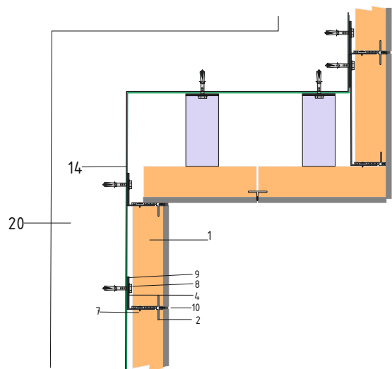
SECCIÓN TRANSVERSAL
